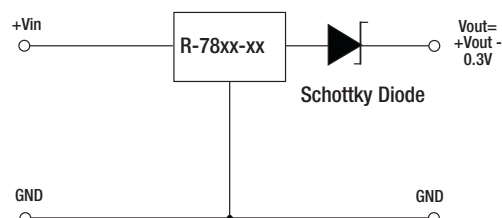
Optional Protection 2:
