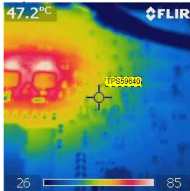
Figure 45. CPU2 IC
