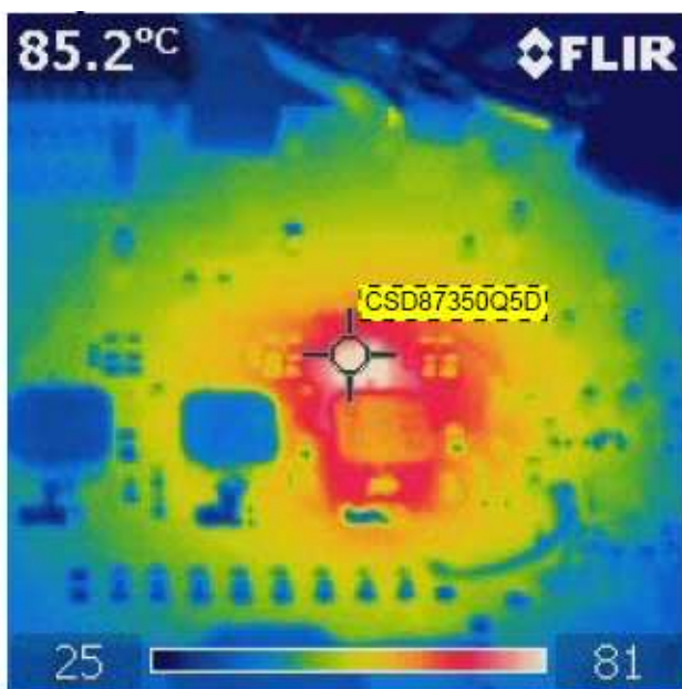
Figure 58. CPU1 MOSFET
