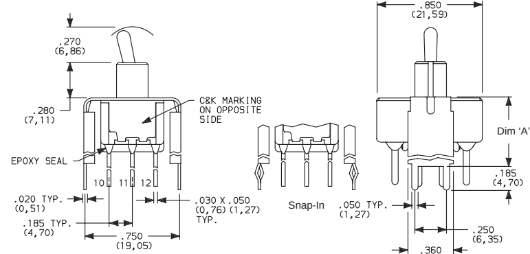
7401MD9_BE 4PDT
