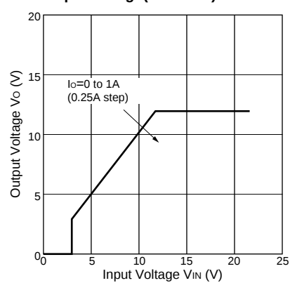
Output Voltage(SI-3123N)
