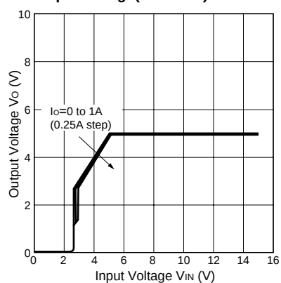
Output Voltage(SI-3053N)
