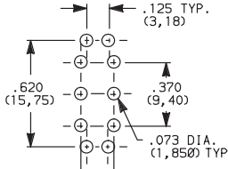
7201J1_BE2 DPDT
