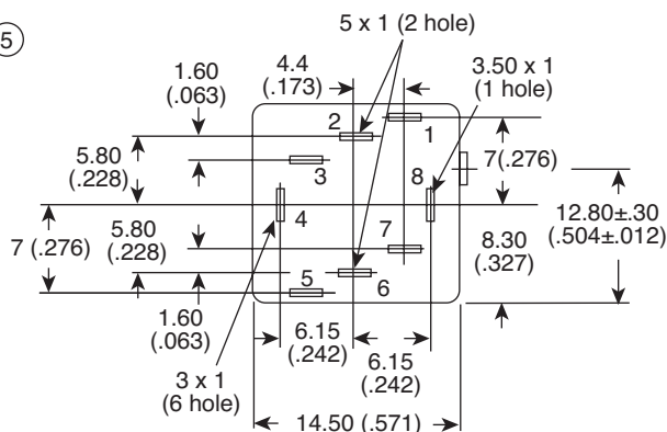
P.C.B. LAYOUT
