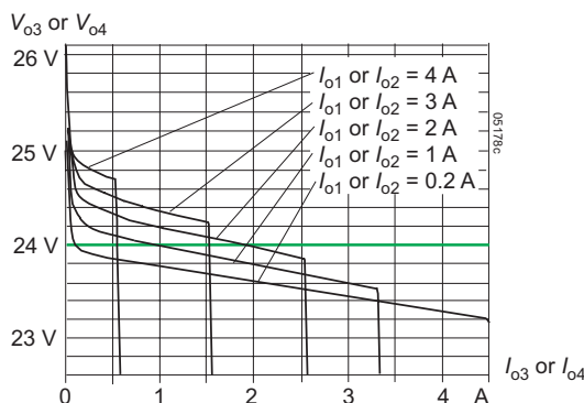
Fig. 16 24 V tracking output V_o = f(I_o) , V_i = V_{i nom}
