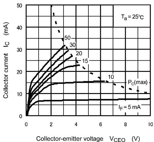
Fig. 11.7 I_C - V_{CEO}
