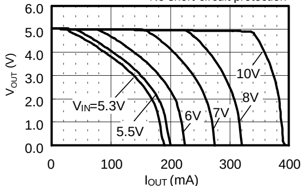
S-812C50A (Ta=25°C)
