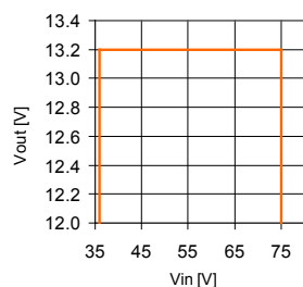
Vin range: 36-75Vdc BMR457xx04/xxx
