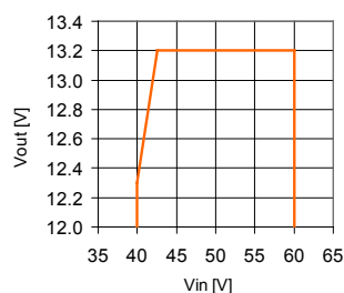
Vin range: 40-60Vdc BMR457xx00/xxx
