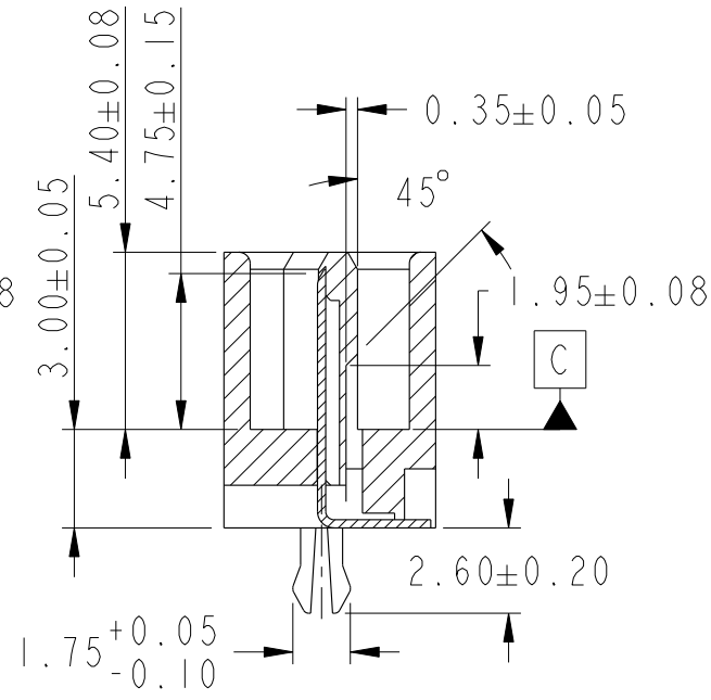
SECTION A-A METAL CLIP D
