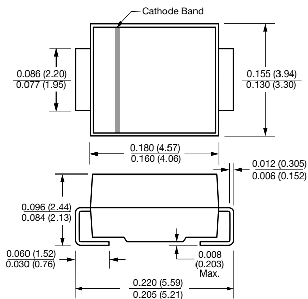
SMB (DO-214AA)
