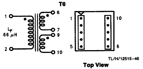
FIGURE 28. Schott 67140900
