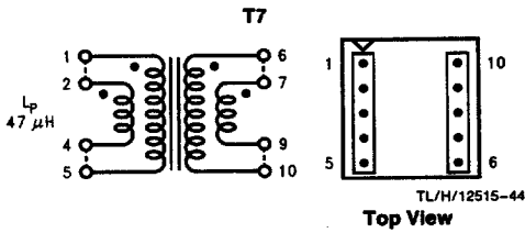
FIGURE 27. Schott 25606
