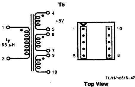
FIGURE 29. Schott 67140890
