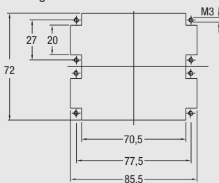
Montageausschnitt/Panel cut-out
