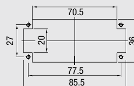
Montageausschnitt Panel cut-out
