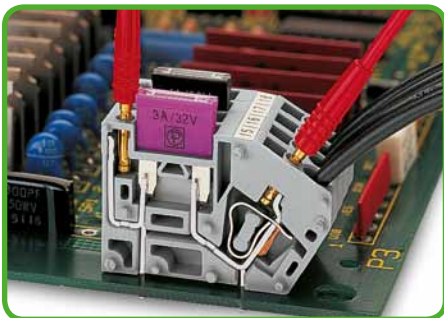
Prüfen - Sicherungsklemme
