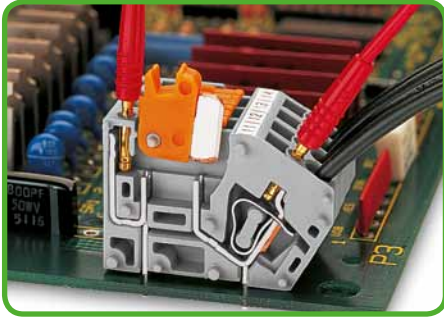
Prüfen - Trenn- und Messklemme
