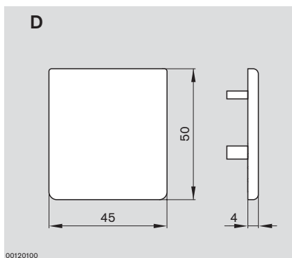
Cap
