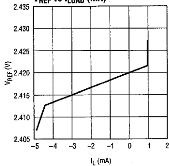
VREF vs ILOAD (mA)
