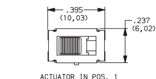
ACTUATOR IN POS. 1
