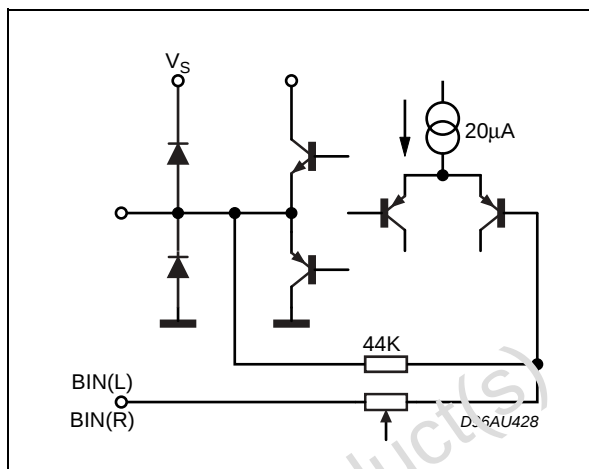
Figure 30. PIN: 20
