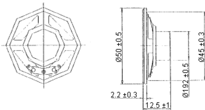
Dimensions : Millimetres
