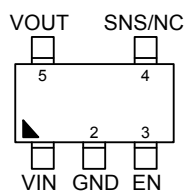
TSOT-23-5
