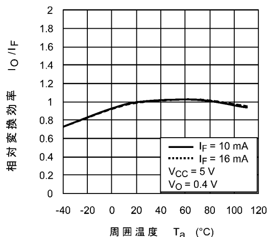
図 12.2.8 I_O/I_F - T_a
