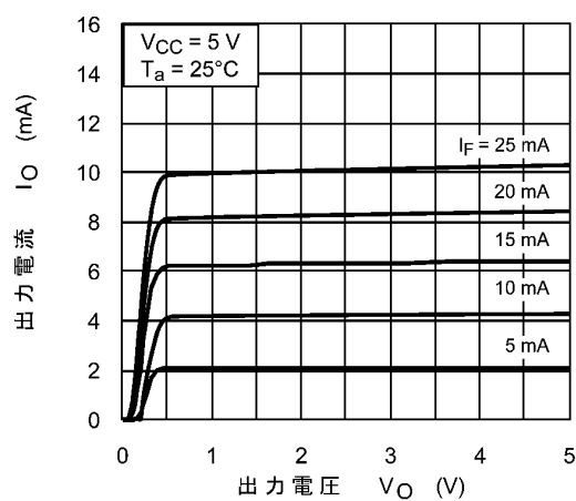
図 12.2.11 I_O - V_O
