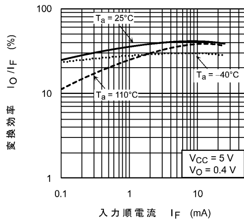
図 12.2.4 I_O/I_F - I_F
