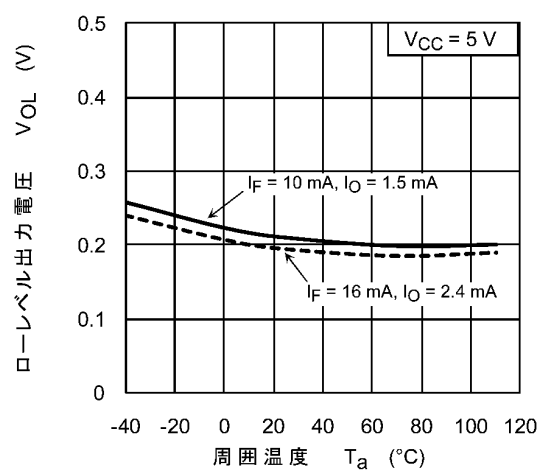
図 12.2.15 V_{OL} - T_a
