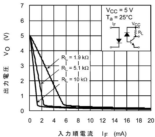
図 12.2.13 V_O - I_F
