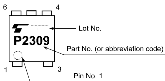
図 15.1 現品表示
