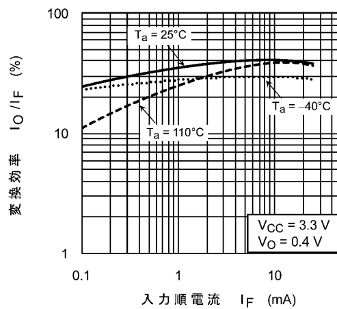
図 12.2.6 I_O/I_F - I_F
