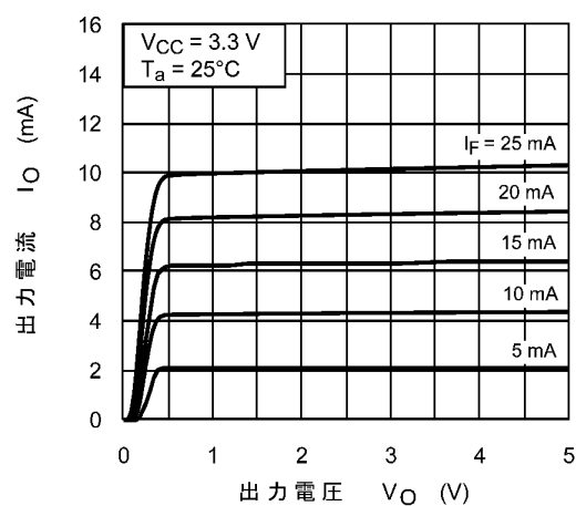
図 12.2.12 I_O - V_O
