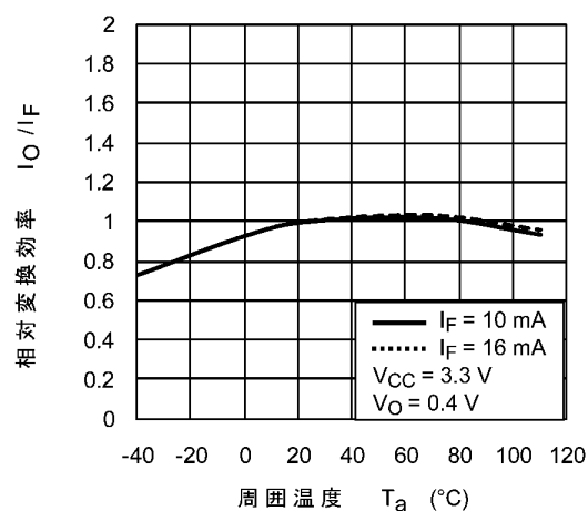
図 12.2.10 I_O/I_F - T_a
