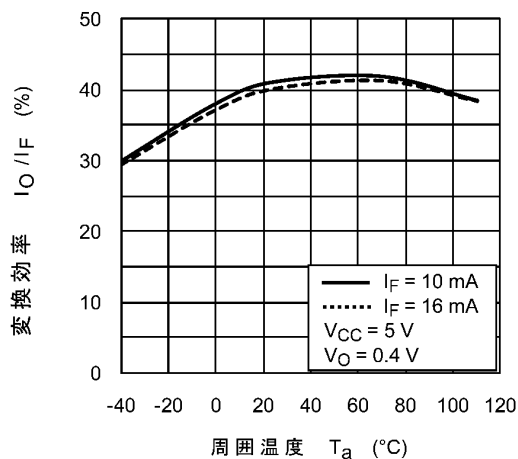
図 12.2.7 I_O/I_F - T_a
