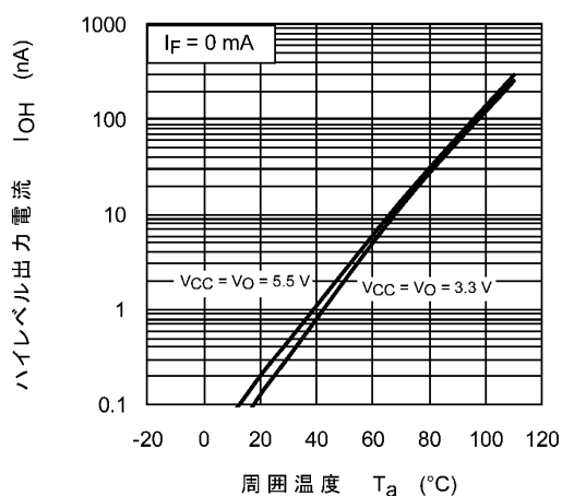
図 12.2.2 I_{OH} - T_a
