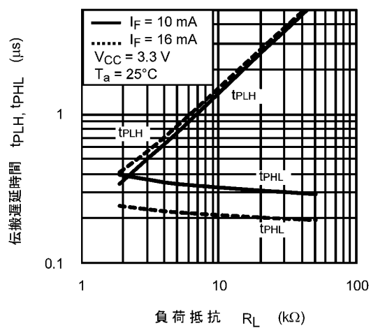
図 12.2.20 t_{PLH} , t_{PHL} - R_L
