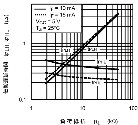
図 12.2.19 t_{PLH} , t_{PHL} - R_L
