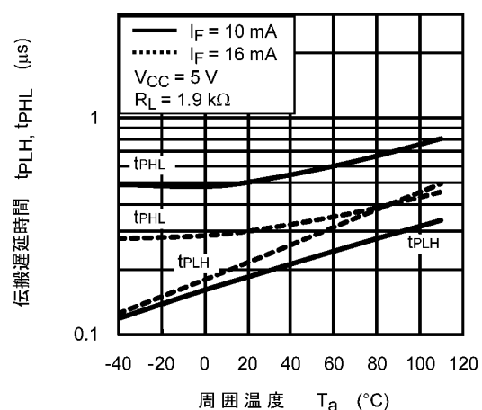
図 12.2.17 t_{PLH}, t_{PHL} - T_a
