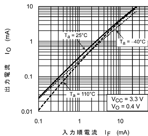
図 12.2.5 I_O - I_F
