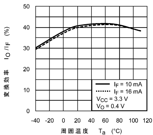
図 12.2.9 I_O/I_F - T_a
