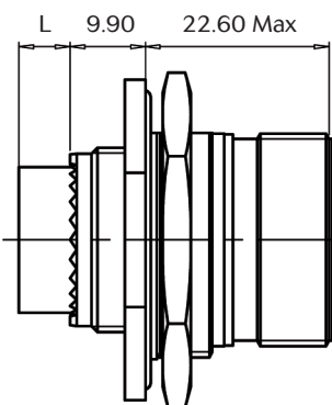
Type 7 Jam Nut Receptacle
