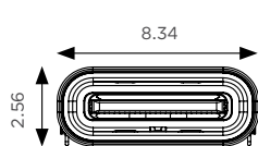
USB TYPE-C
