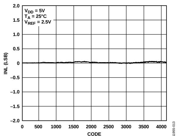
Figure 13. AD5681R INL
