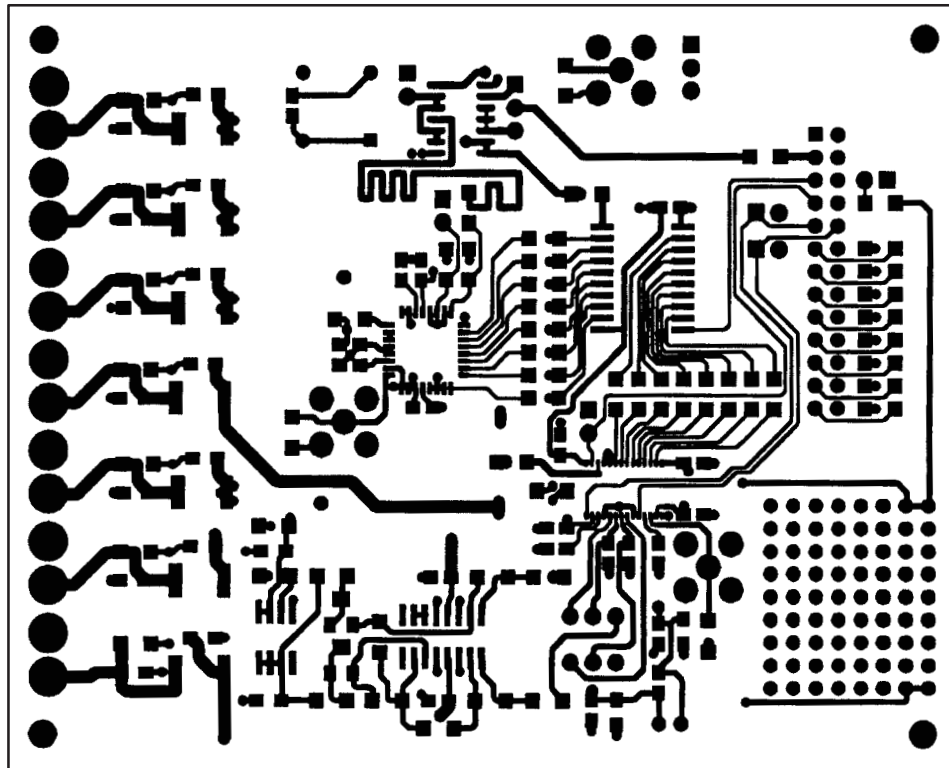
Top Layer
