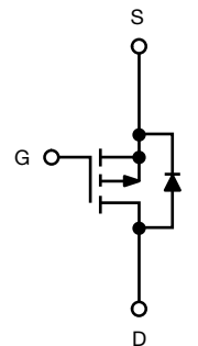
P-Channel MOSFET
