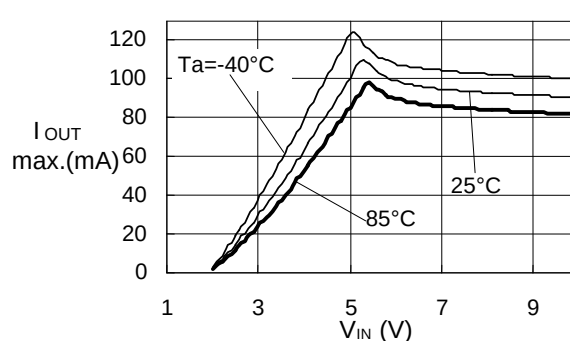
S-817A50A
