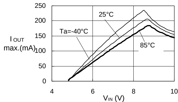
S-817A50A
