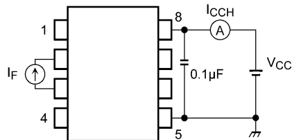
Fig. 12.1.3 V_{OH} Test Circuit
