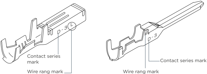
Receptacle Contact
