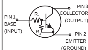
SC-70 / SOT-323
