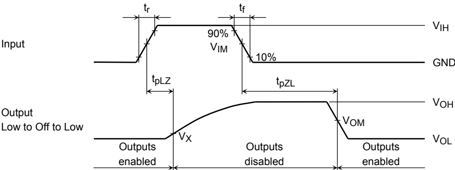
図 2 tpLZ, tpZL
