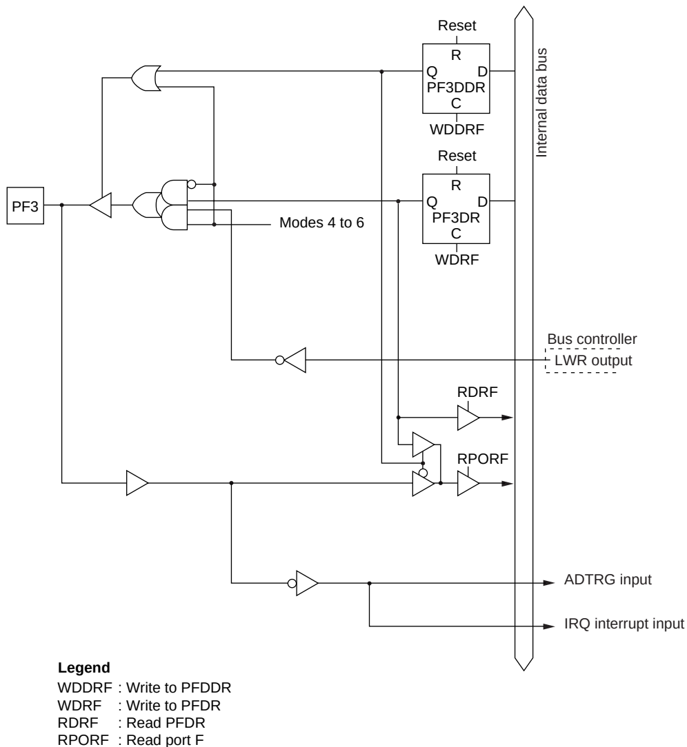
Figure C-23 (d) Port F Block Diagram (Pin PF3)
