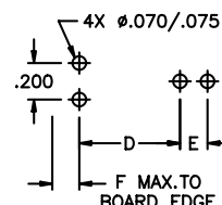
P.C. LAYOUT
