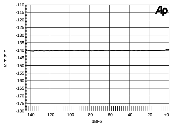
48 kHz:44.1 kHz
