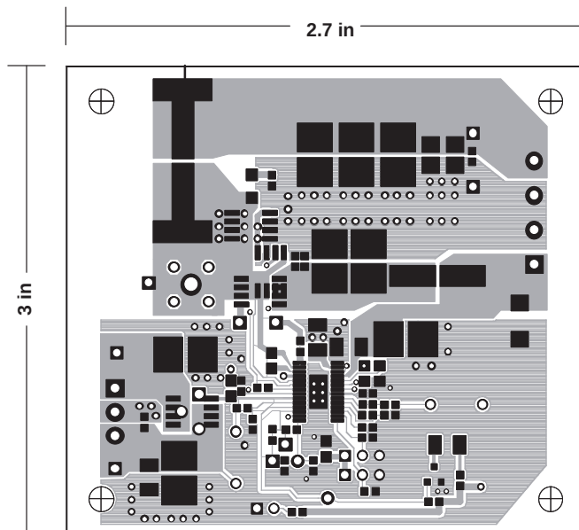
Figure 29. Top Layer
