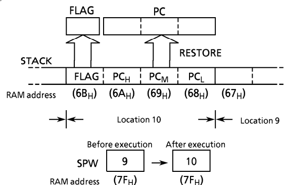
(d) At execution of the interrupt return instruction
