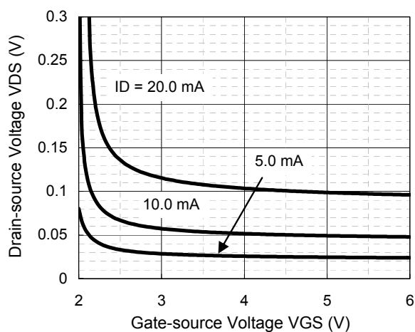
VDS - VGS
