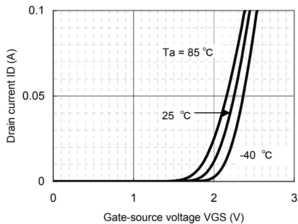
ID - VGS
