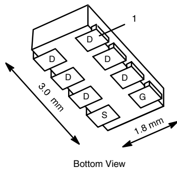
1206-8 ChipFET®
