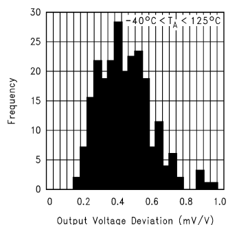
Thermal Hysteresis
