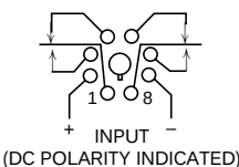
Fig. 1 8 Pin
