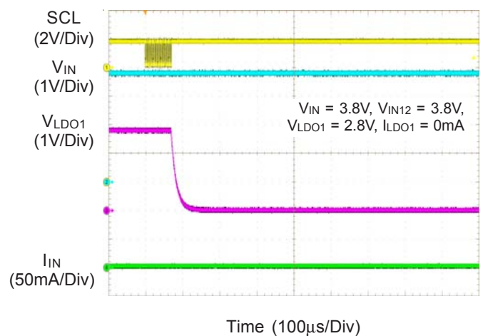
LDO1 Power Off
