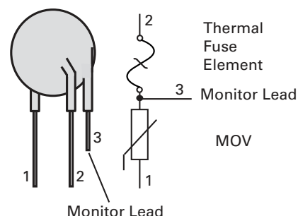
iTMOV® Varistor
