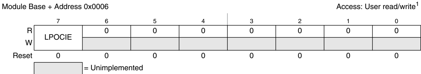
Figure 15-8. LIN Interrupt Enable Register (LPIE)
