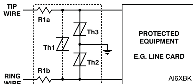
Protection Module
