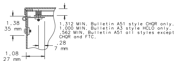
DETAIL Y
