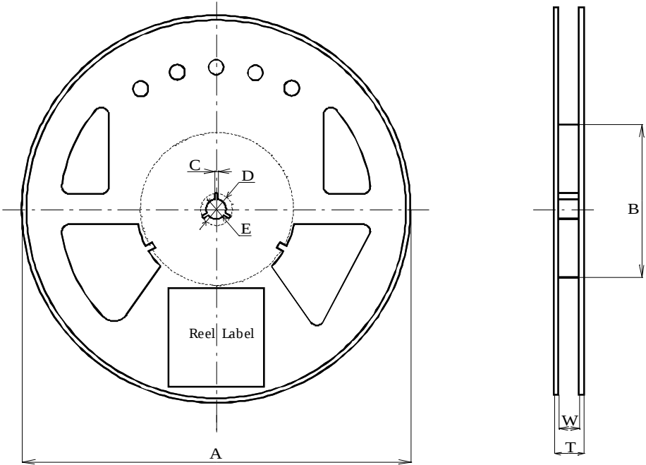
第3図 プラスチックエンボステープの外形寸法図 Figure 3. Dimensions of Plastic Embossed Tape
