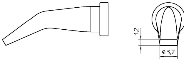
LT MX2 Lötspitze 3,2mm
