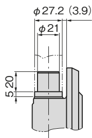
ジョイントA Joint A (φ27.2パイプ用) (For φ27.2 pipe)
