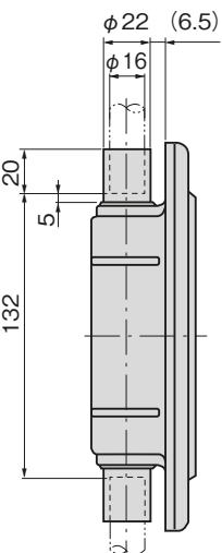
ジョイントC Joint C (φ16丸棒用) (For φ16 round rod)
