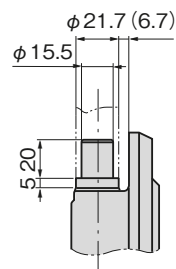
ジョイントB Joint B (φ21.7パイプ用) (For φ21.7 pipe)
