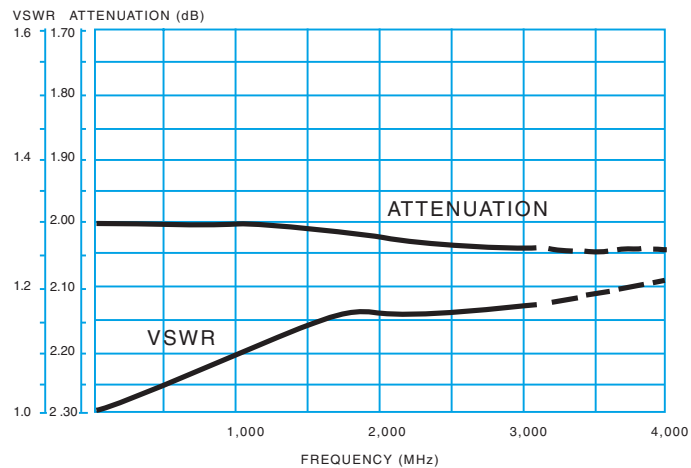
2 dB ATTENUATOR
