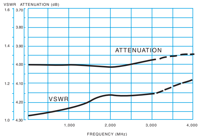
4 dB ATTENUATOR
