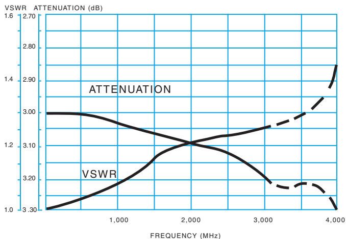
3 dB ATTENUATOR
