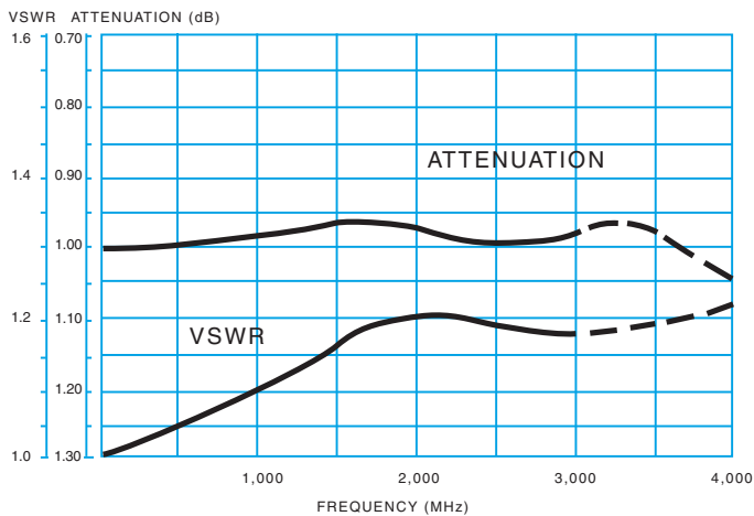
1 dB ATTENUATOR
